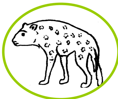
Höhlenhyäne
