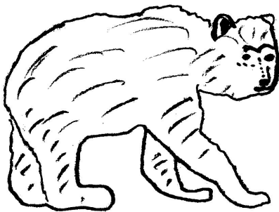
Höhlenbär
