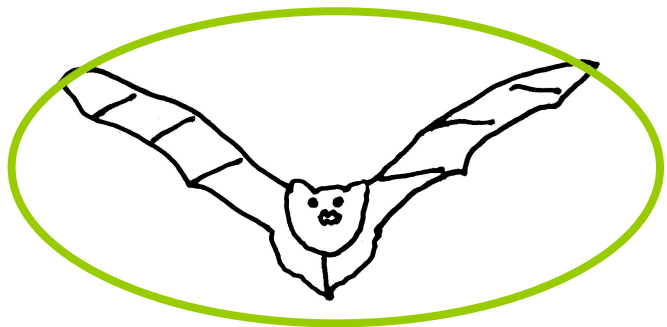
Fledermaus
