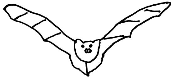
Fledermaus
