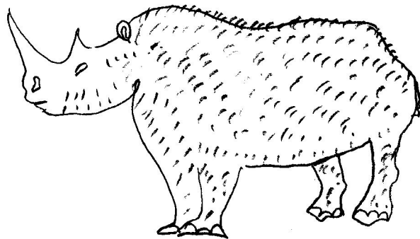
Wollnashorn
