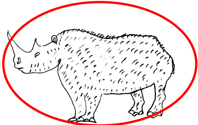
Wollnashorn
