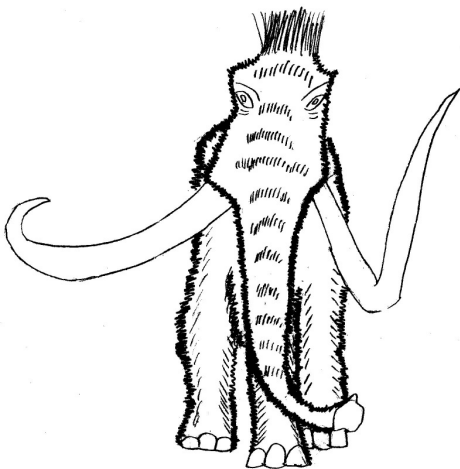
Mammut
