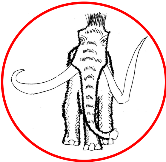
Mammut
